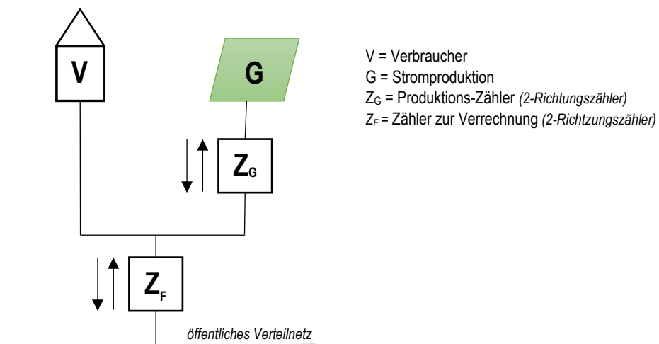
Beispiel Messung nach Eigenverbrauchsprinzip - Stromerzeugungsanlage über 30 kVA → Reihe 3
