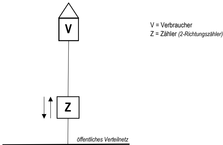
Beispiel Messung nach Eigenverbrauchsprinzip - Stromerzeugungsanlage bis max. 30 kVA 2
