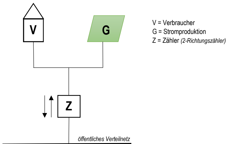
Beispiel Messung nach Eigenverbrauchsprinzip - Stromerzeugungsanlage über 30 kVA → Reihe 3
