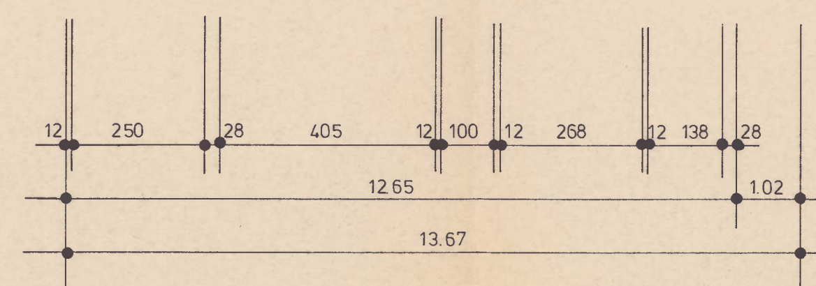
DACHGESCHOSS
