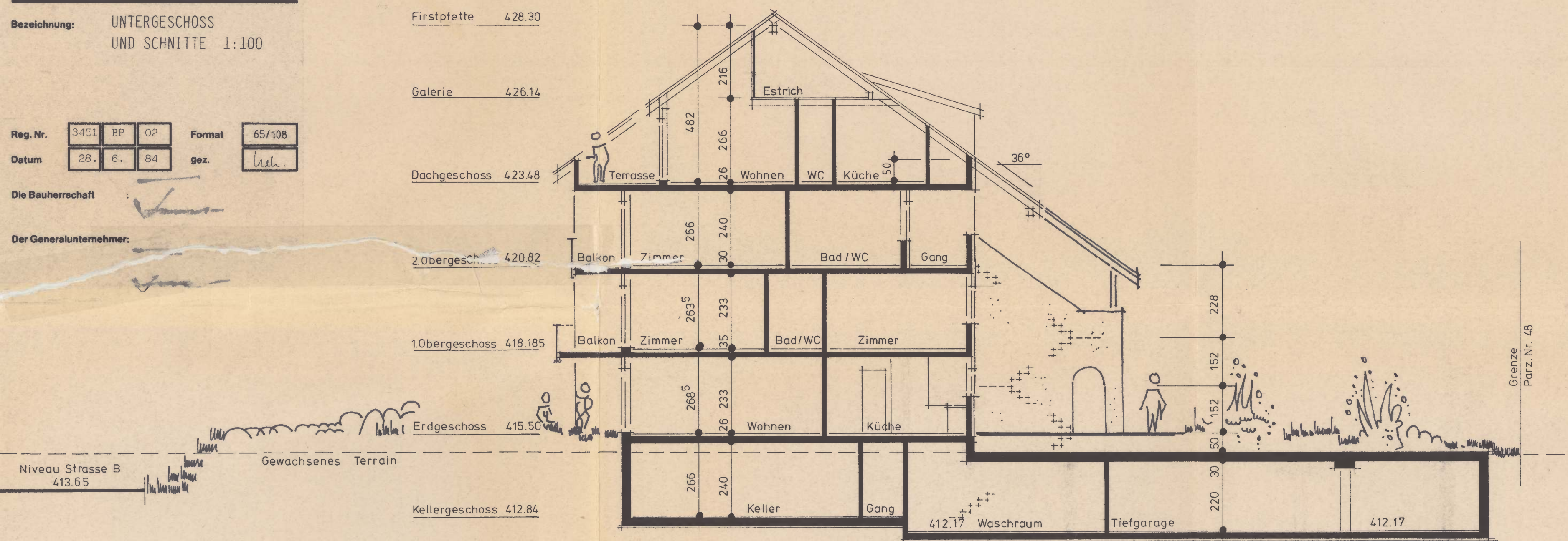
SCHNITT 2-2
