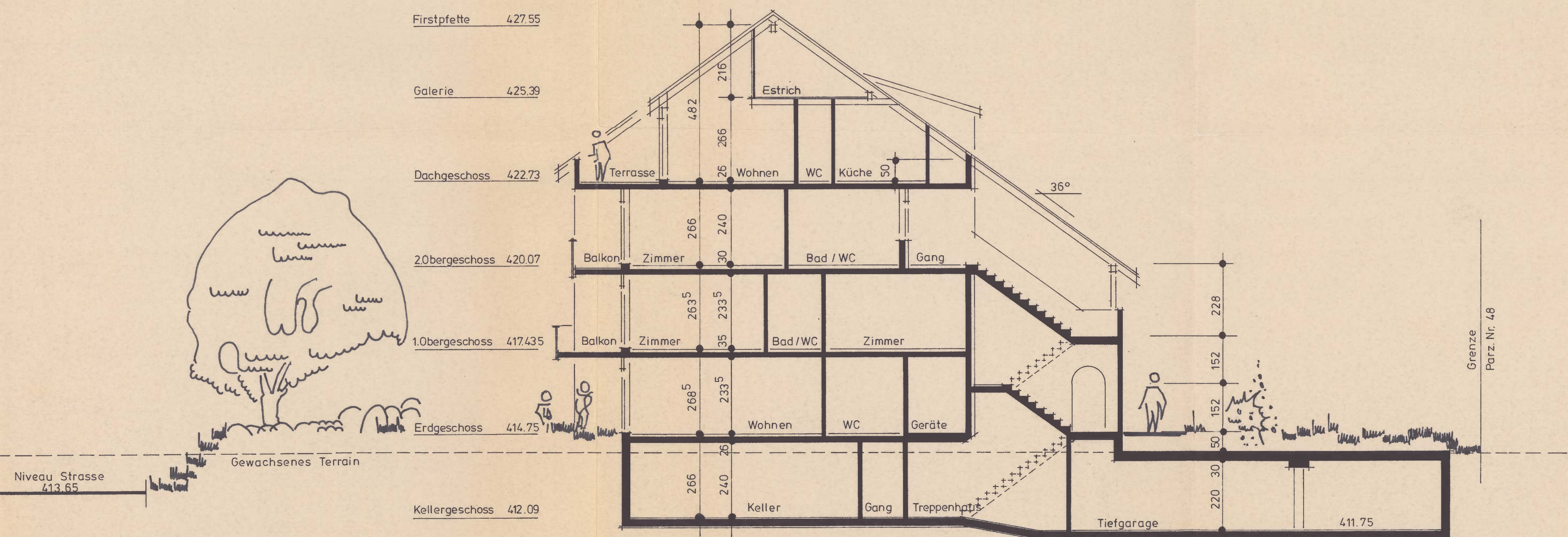
SCHNITT 1-1
